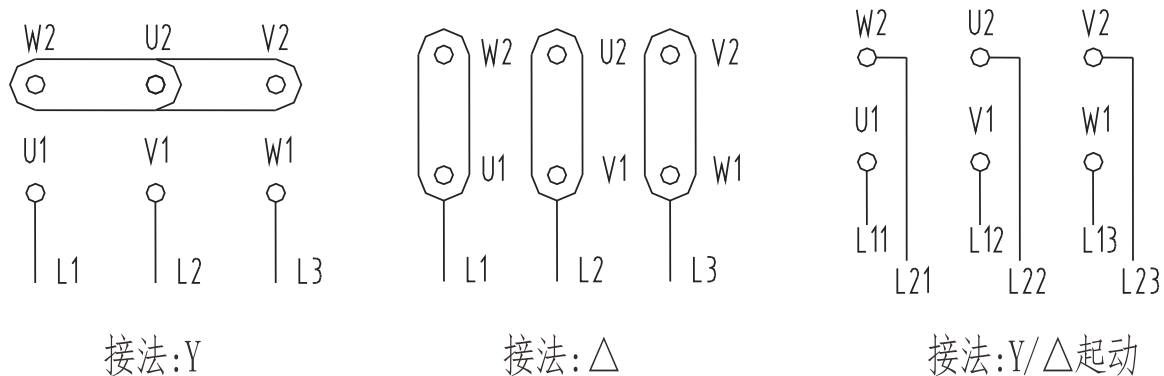
图1.接线指示图 Fig. Wring Diagram
